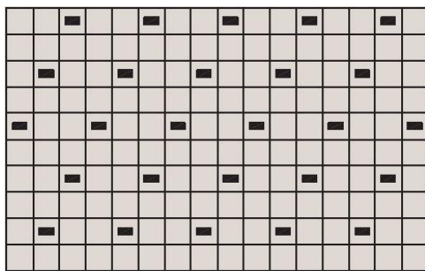
Schema D: Una tegola fermaevne ogni terza tegola in ogni seconda fila
