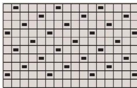
Schema E: Una tegola fermaeve ogni quinta tegola Scheme E: 1 snow stop tile every 5th tile on every row
