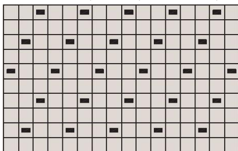
Schema D: Una tegola fermaneve ogni terza tegola in ogni seconda fila Scheme D: 1 snow stop tile every 3 th tile on every 2 nd row
